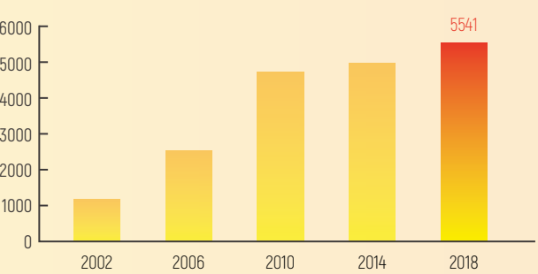
2002年-2018年发电量 (单位:亿千瓦时)
